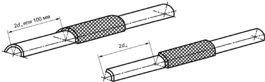
Рисунок ДА.1 - Подготовка испытуемых образцов
