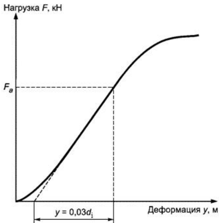
Рисунок В.1 - Кривая "нагрузка-деформация"
